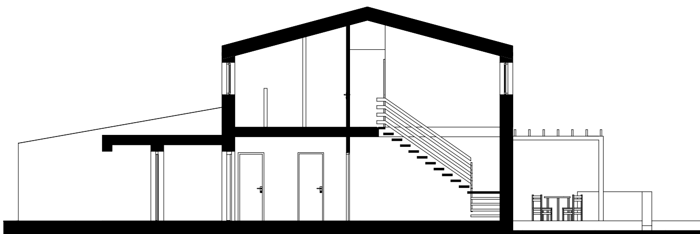
■ ■ ŘEZ_1:120
