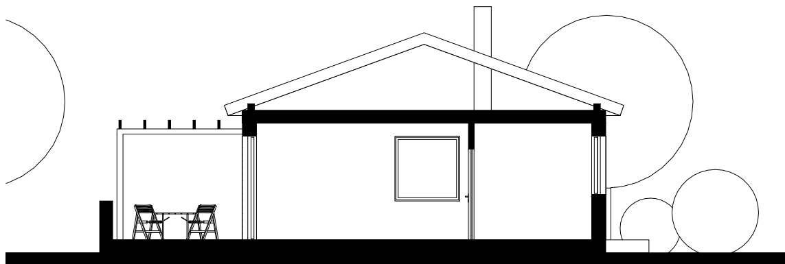
■ ■ ŘEZ_1:120
